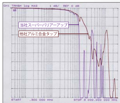
100MHzから一気にノイズ減衰に成功している。効果的に高周波ノイズを誘導していると言える。
